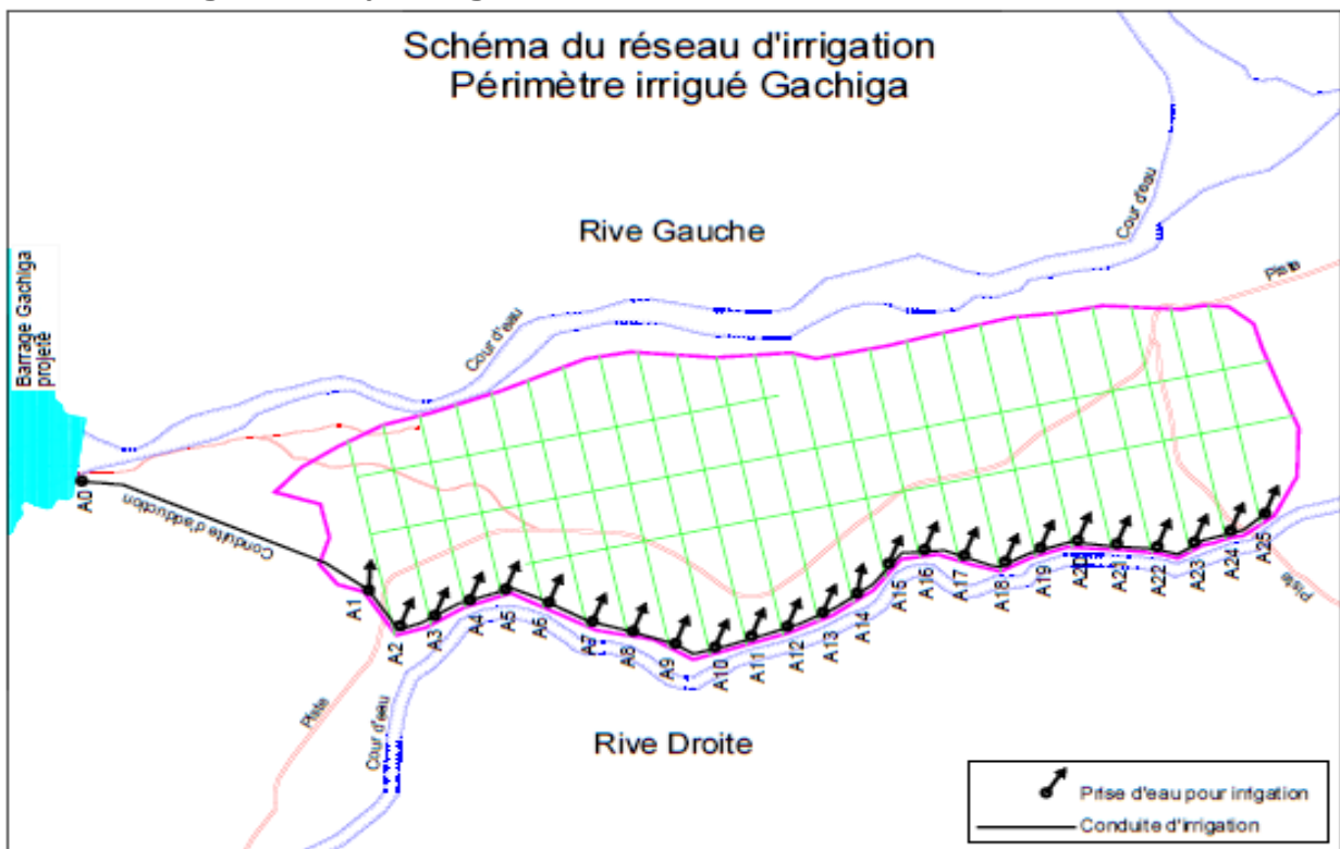
Figure 9 : Schéma du réseau d'irrigation – Périmètre irrigué de Barkéhi (Gaschiga)
