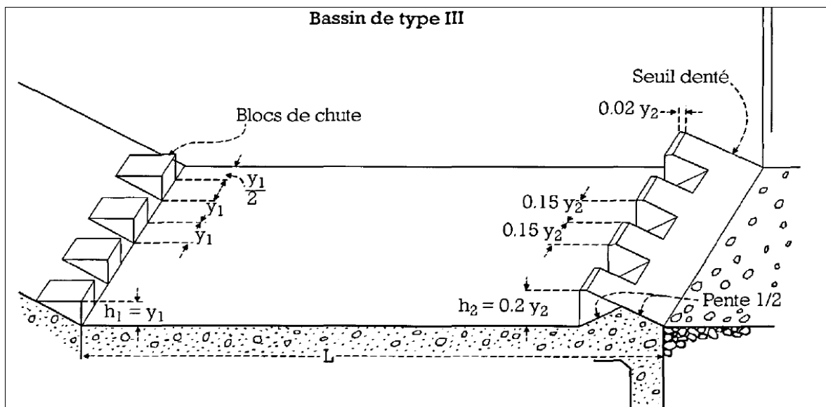
Figure 7 : Schéma du bassin de dissipation « type 3 »
