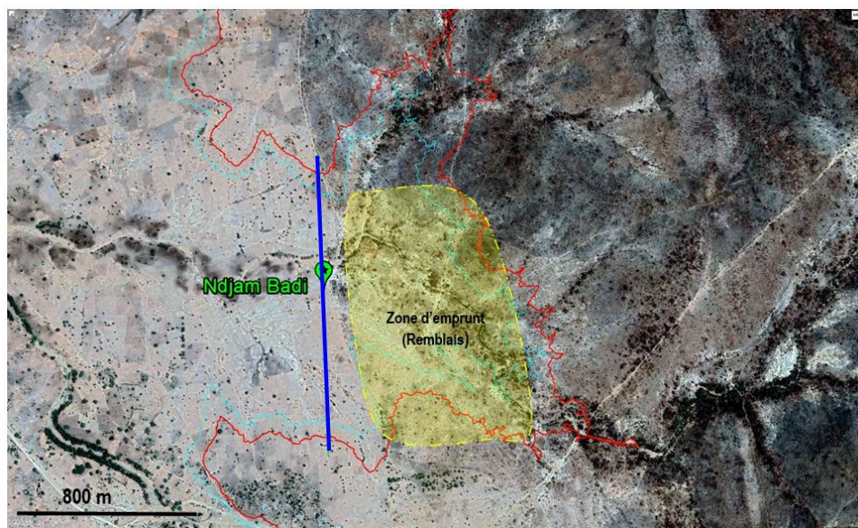
Localisation de la zone d'emprunt du site de Ndjam-Badi (Source : COMETE)
